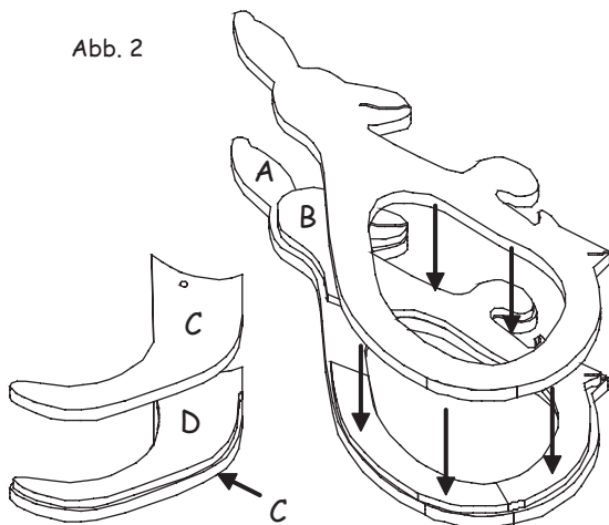
Zusammenleimen
