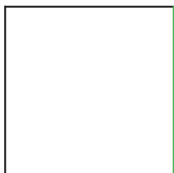
vierkant
