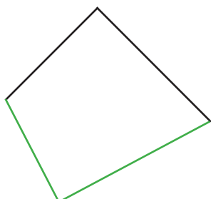
onregelmatige veelhoek
