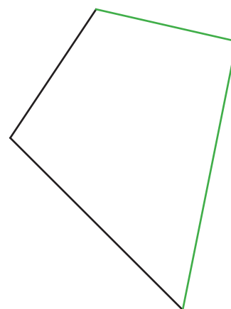
onregelmatige veelhoek
