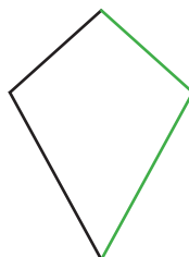
vlieger
